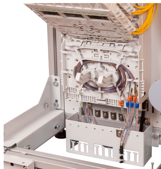
Vláknový organizér (Subrack B)
