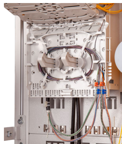
Vláknový organizér (Subrack A)
