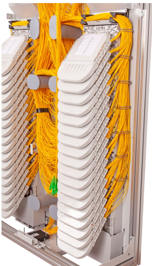
Výstup patchcordů z kazet KM 5
