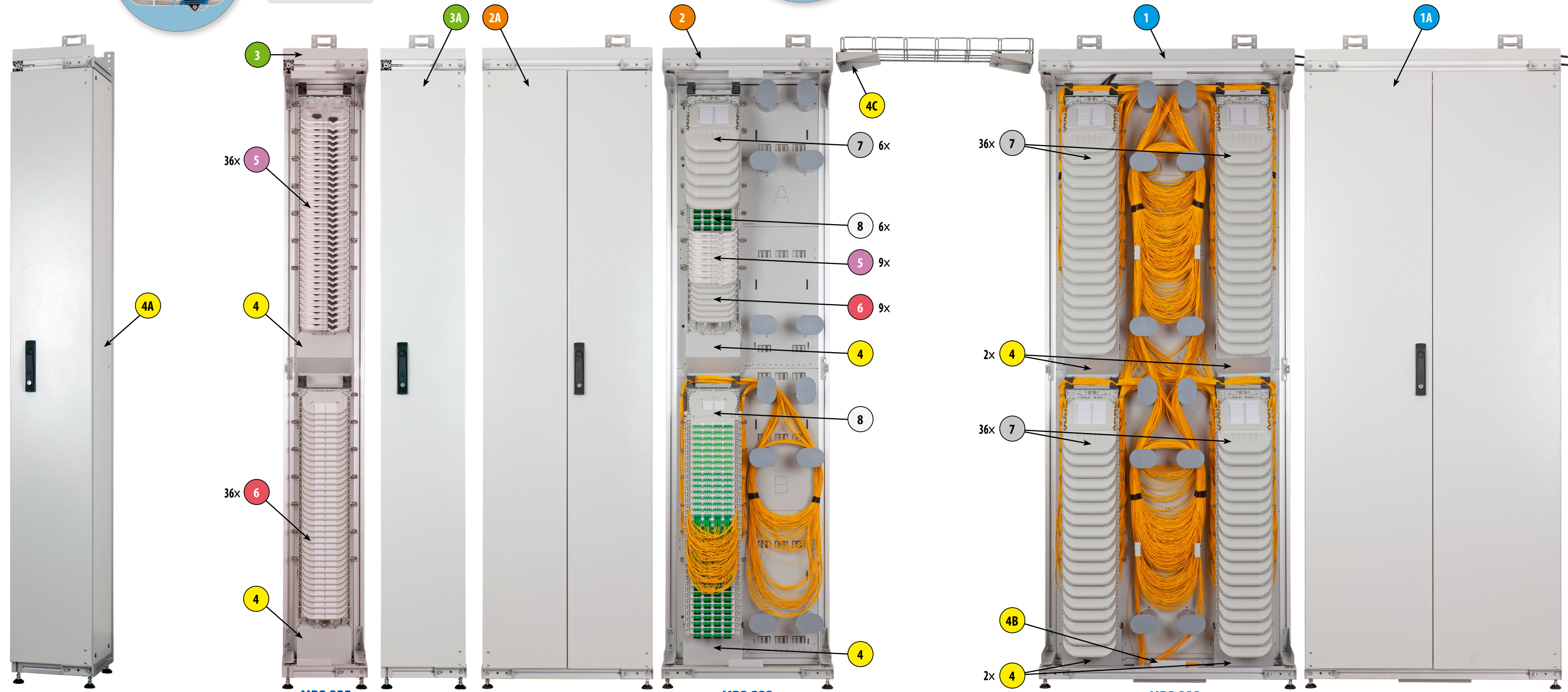
MDO 300 Kapacita až 1 728 svárů, 576x SC / 1152x LC konektor (bez vyvazovací části)
