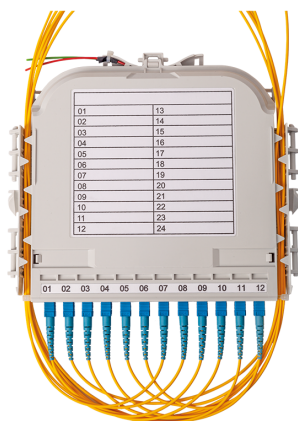
KM 5 (s víkem a samolepkou)
