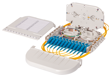
Optická kazeta KM 5 (set)
