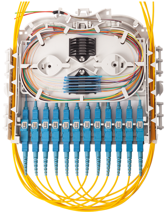
Optická kazeta KM 5
