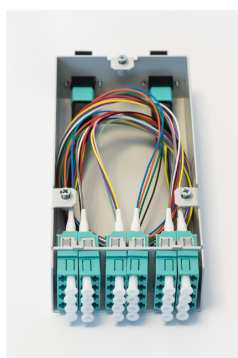
Modul 6x LCQ MPO – OM3 předvystrojený
