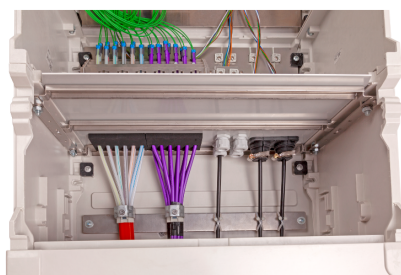
Pilřový optický rozvaděč MDP OZ 144/288
