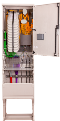
Pilřový optický rozvaděč MDP OZ 144/288
