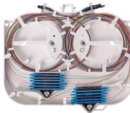
KM 4 (na svařování, až 24 svárů)
