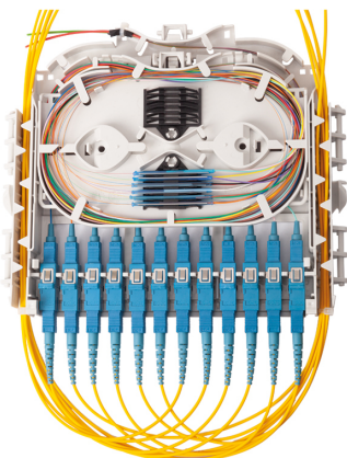
KM 5 (pro adaptéry, až 12× SC / 24× LC konektor, až 24 svárů)
