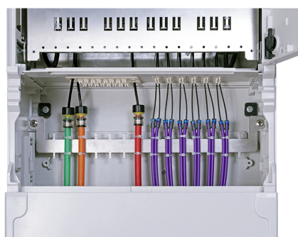
MDP OZ 576S (ukončení)
