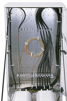
MDP OZ 864S (vedení kabelů na výklopný rám)
