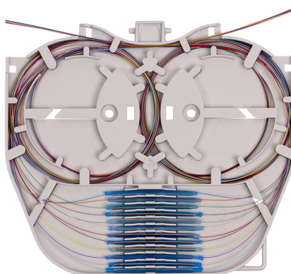
Optická kazeta KM 9 (na svařování, až 12 svárů)
