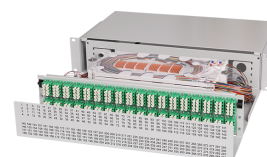
Výsuvná optická vana UHD ORMP 2U 288LC
