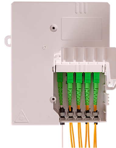
MTeH MINI – Plug & Play Solution – Using Splitter
